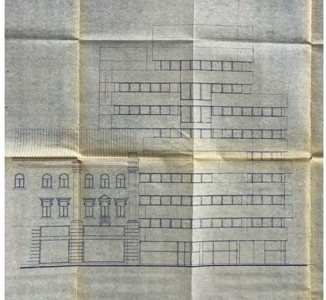
Originalaus projekto dokumentacija 1985 m. Fasadas iš Gedimino pr. pusės
