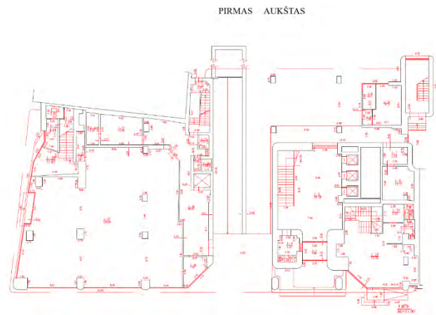
2020 m. 1 aukšto kadastrinis planas
