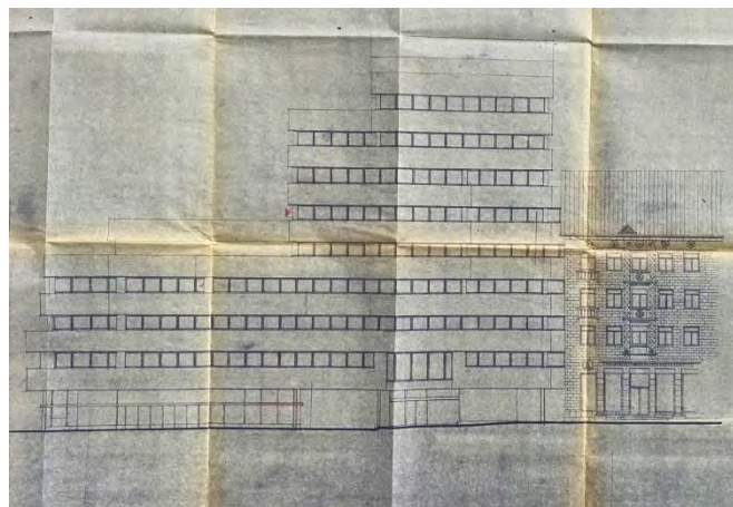
Originalaus projekto dokumentacija 1985 m. Fasadas iš A. Stulginskio g. pusės
