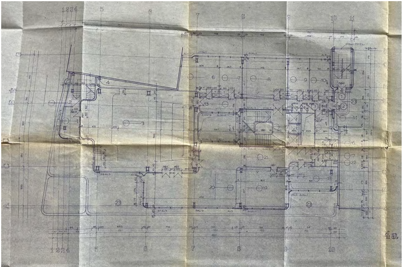
Originalaus projekto dokumentacija 1985 m. 4 aukšto plano brėžinys
