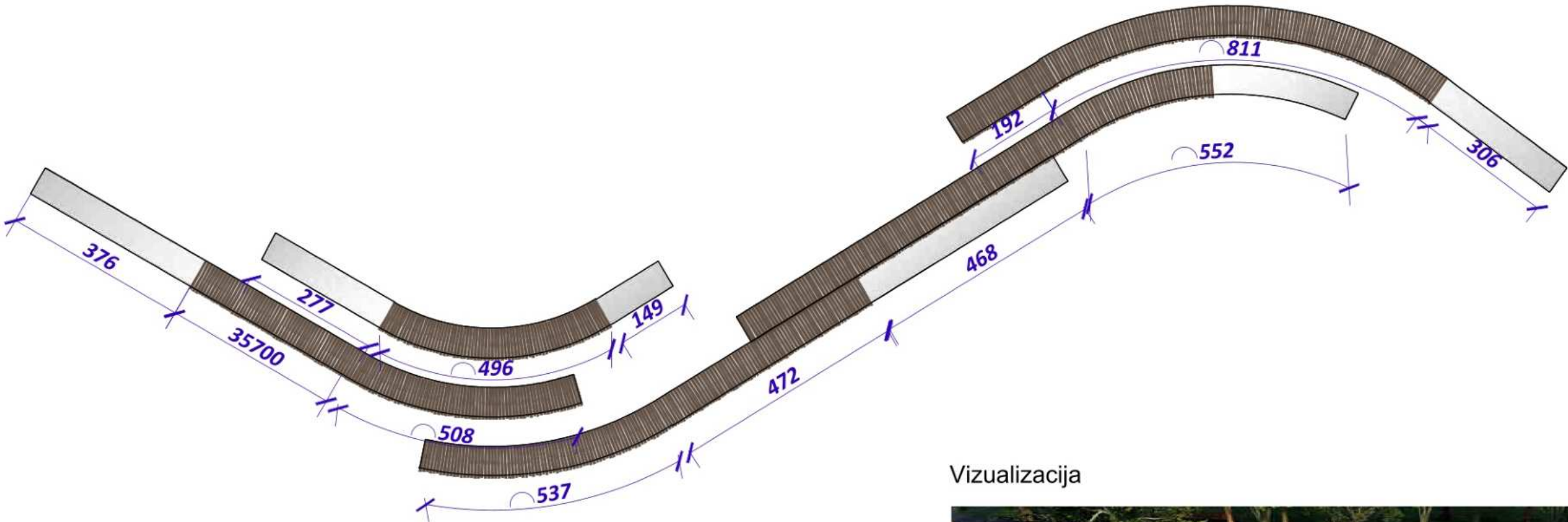
Amfiteatro vaizdas planas M 1:100
