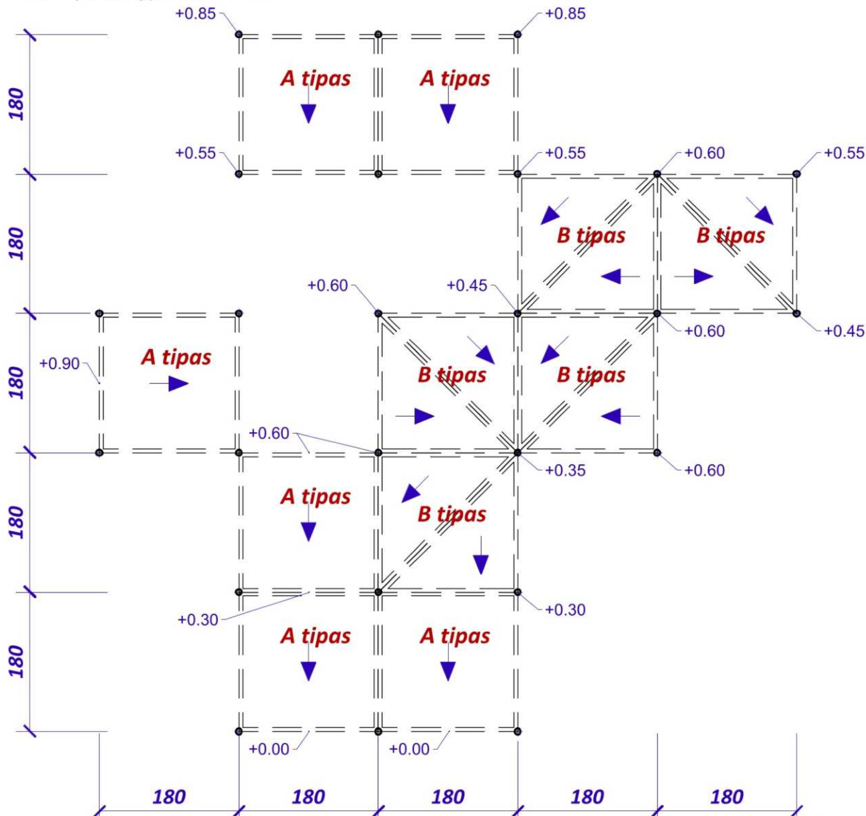
Hamakų atramų planas M 1:50
