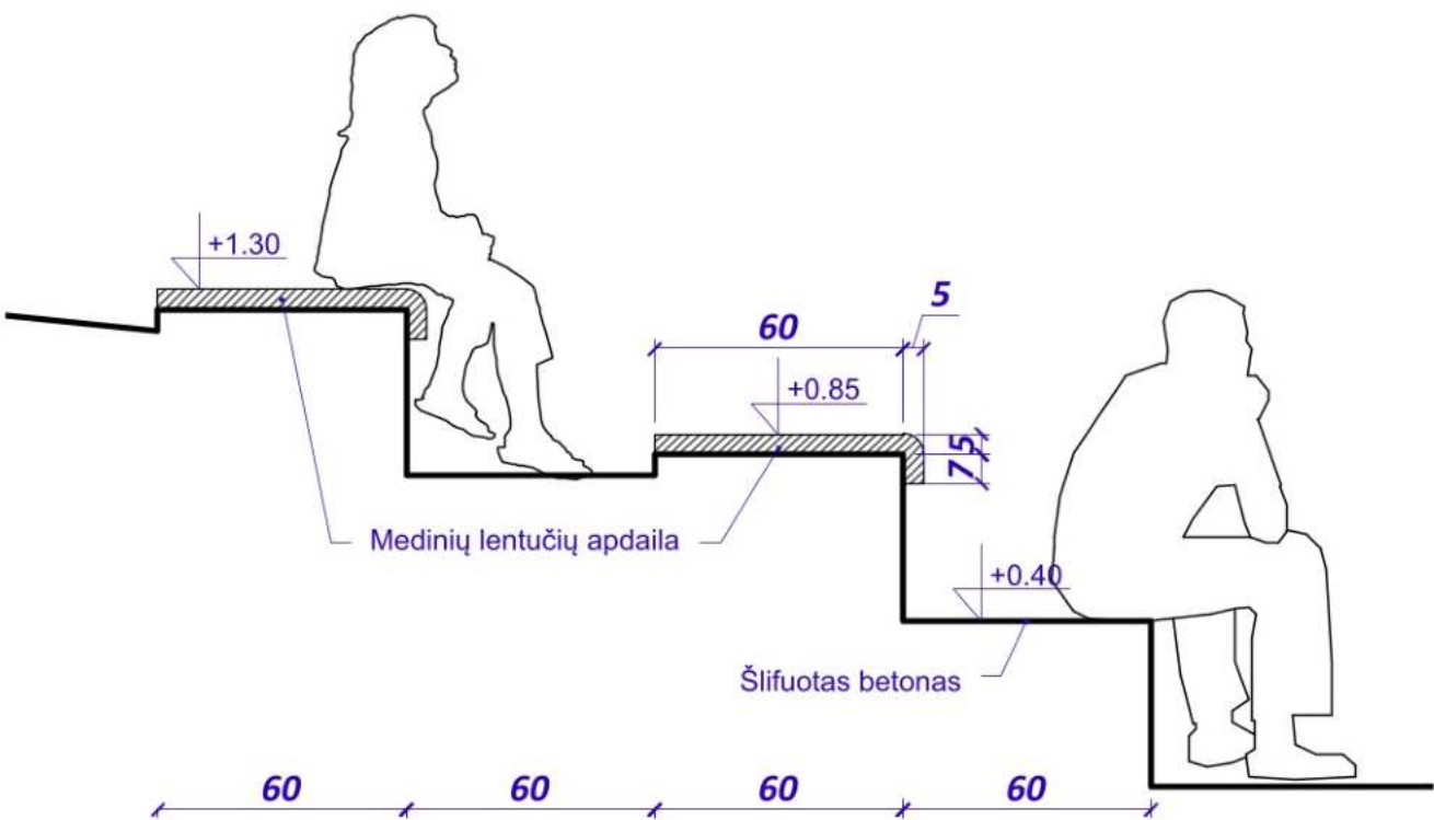
Skersinis pjūvis M 1:20
