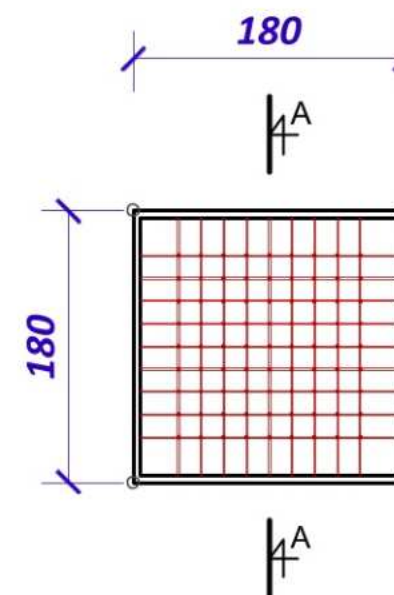
Skersinis pjūvis A-A M 1:50
