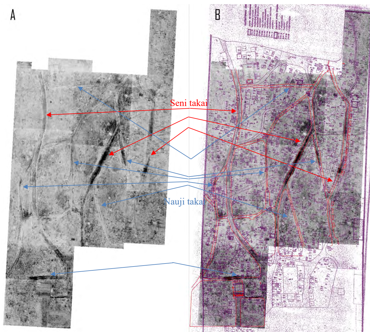
4 pav. Suminis 00-10 ns anomalijų žemėlapis (0 – 60 cm gylio). Sumuotas georadaro plokštuminis pjūvis (A), Suminis georadaro plokštuminis pjūvis su senu kapinių planu ir dabartiniais parko takais pažymėtais raudona spalva (B). Raudonomis rodyklėmis parodyti dabartiniai takai sutampantys su senais kapinių takais, mėlynomis rodyklėmis parodyti nauji takai.
