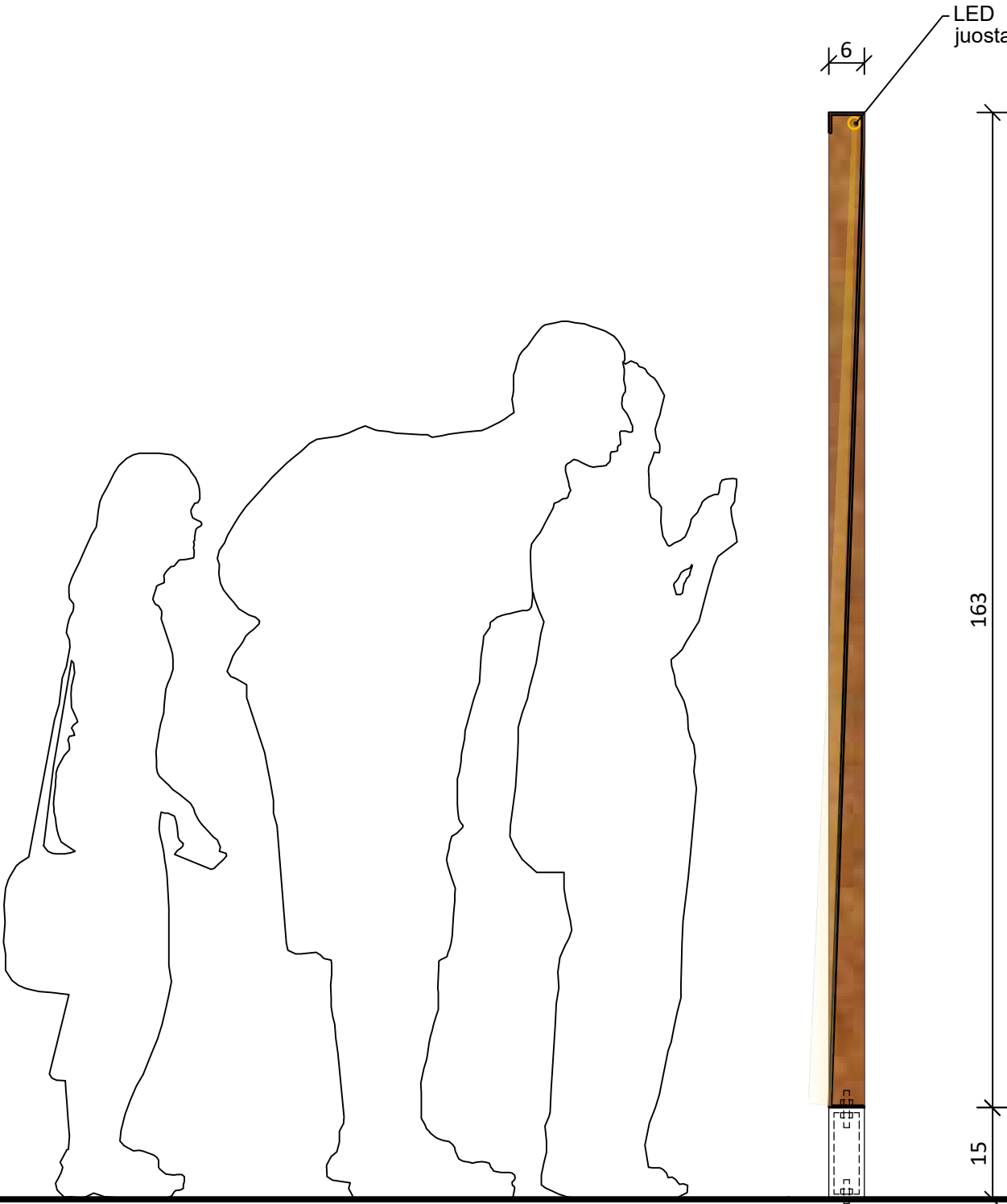
IŠILGINIS PJŪVIS PER STENDA M 1:10
