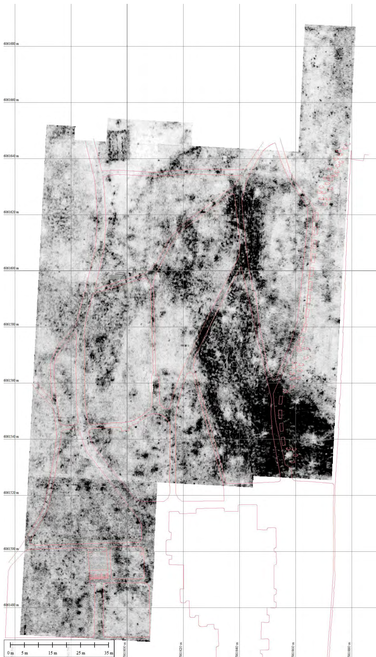
7 priedas. Suminis 30-40 ns anomalijų žemėlapis (180 – 240 cm gylio)
