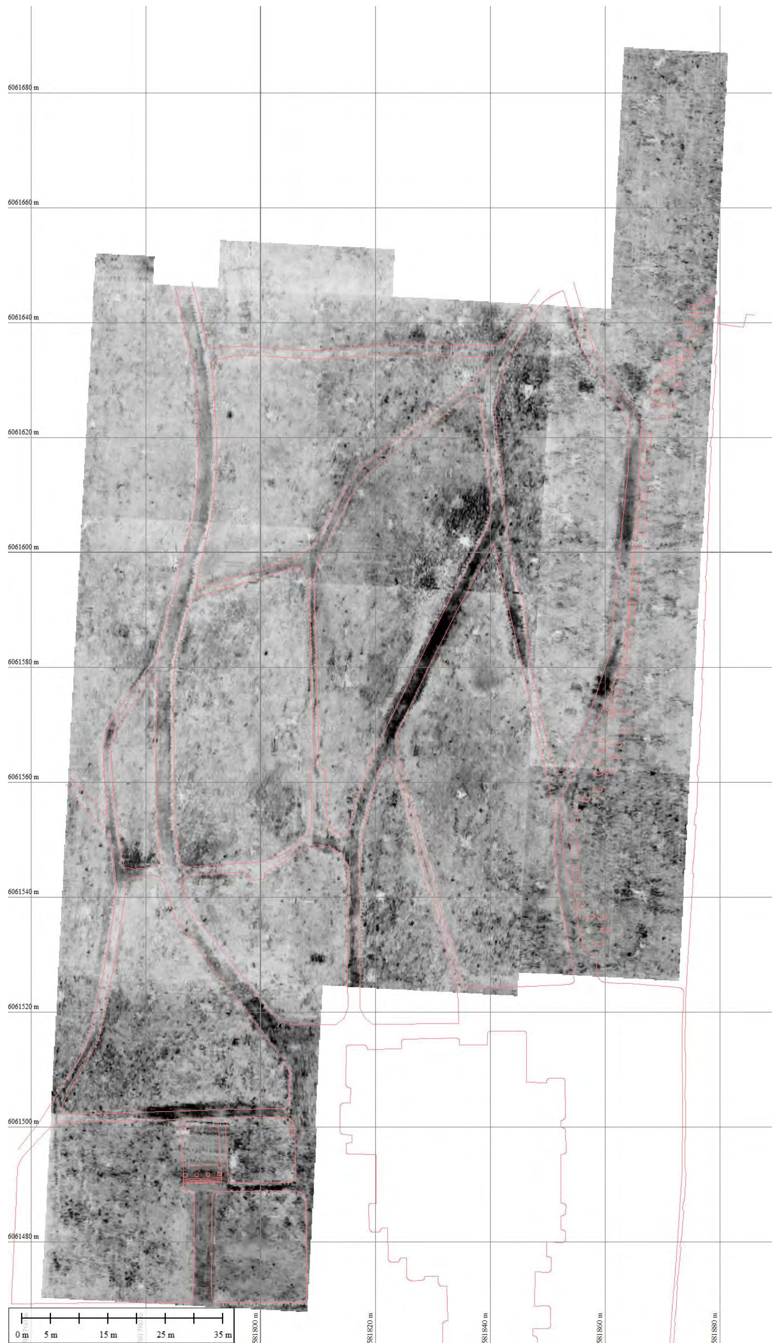
2 priedas. Suminis 00-10 ns anomalijų žemėlapis (0 – 60 cm gylio)
