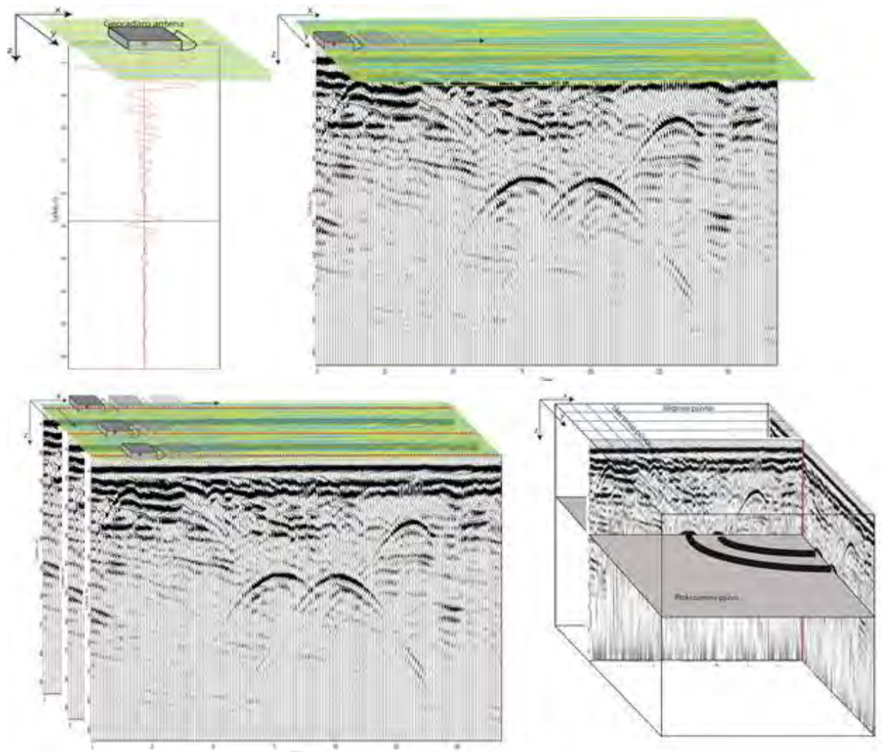
1 pav. Tyrimų georadaru metodika: a) taškinis matavimas; b) profiliniai (2D) tyrimai; c) erdviniai (3D) tyrimai; d) 3D tyrimų masivo vaizdavimas ir plokštuminis pjūvis.
