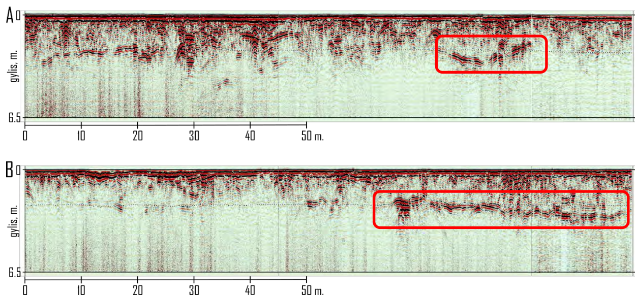
9 pav. Skersiniai pjūviai. A – 91, B - 329. Skersiniuose pjūviuose aiškiai matosi geologiniai sluoksniai.
