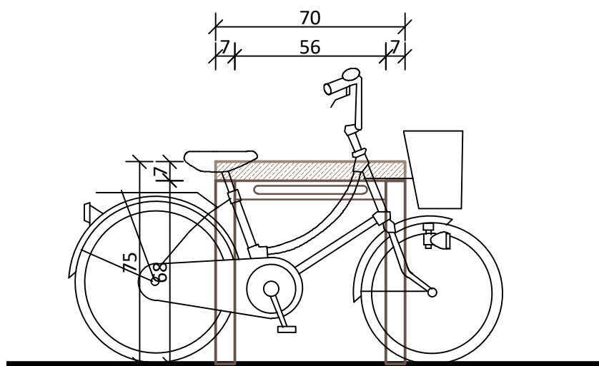
VAIZDAS IŠ PRIEKIO M 1:20
