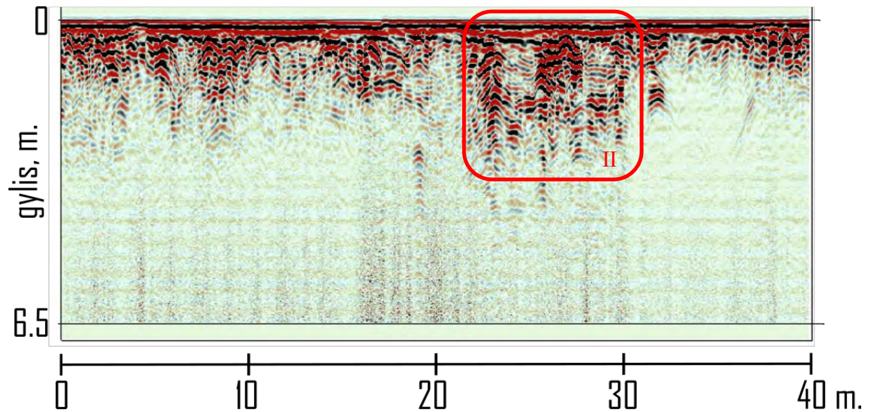
6 pav. Skersinis pjūvis 123-9. Raudonai pažymėta mauzoliejaus pamatų sukelta anomalija.
