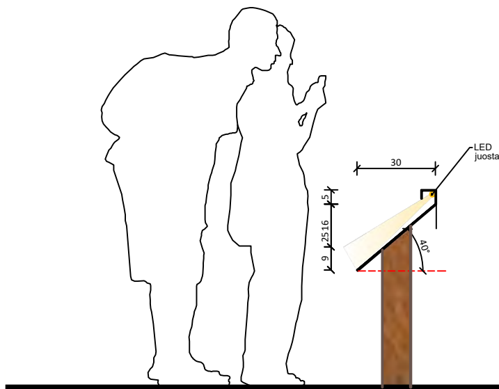
SKERSINIS PJŪVIS M 1:20
