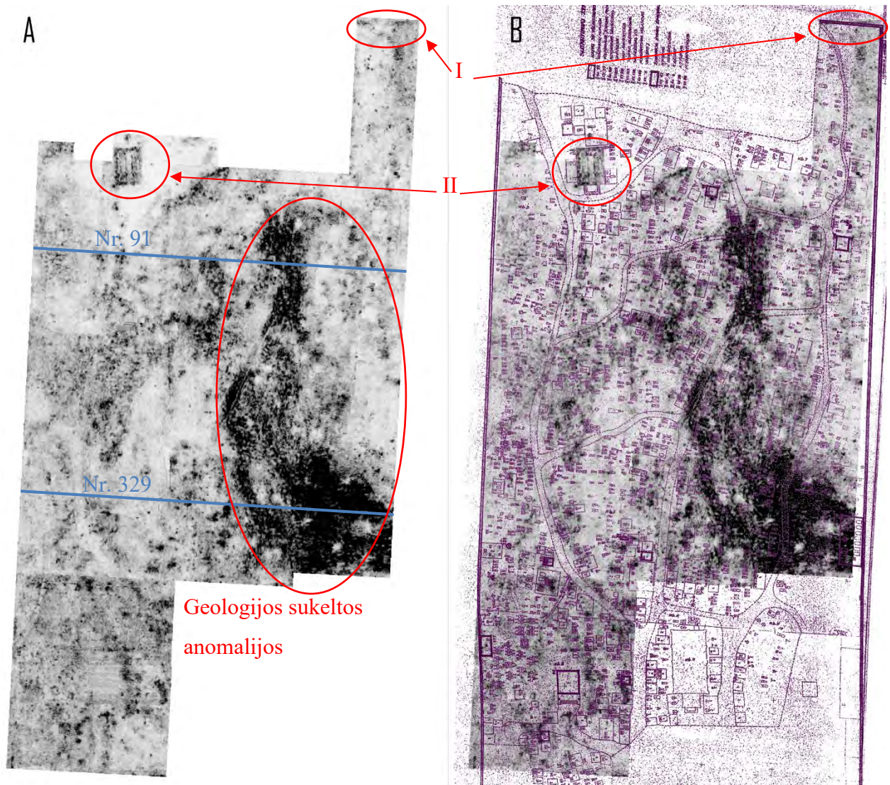
8 pav. Suminis 30-40 ns anomalijų žemėlapis (180 – 240 cm gylio). Sumuotas georadaro plokštuminis pjūvis (A), Suminis georadaro plokštuminis pjūvis su senu kapinių planu (B), raudona spalva pažymėtos anomalijos. Mėlyna spalva pažymėti skersiniai georadaro pjūviai.
