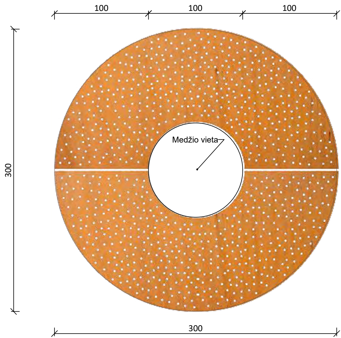
VAIZDAS IŠ VIRŠAUS M 1:20
