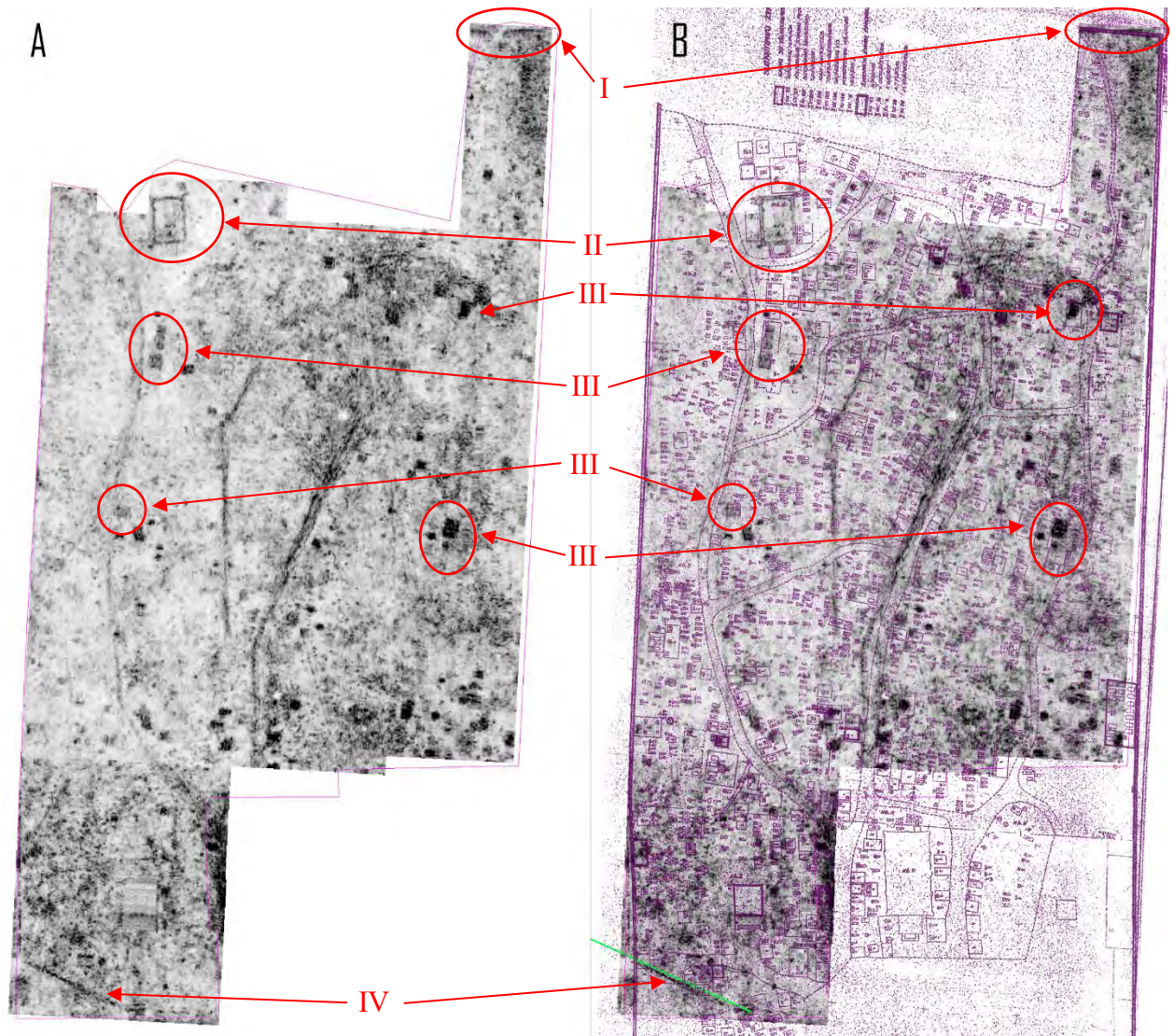
5 pav. Suminis 10-20 ns anomalijų žemėlapis (60 – 120 cm gylio). ). Sumuotas georadaro plokštuminis pjūvis (A), Suminis georadaro plokštuminis pjūvis su senu kapinių planu (B), raudona spalva pažymėtos anomalijos.
