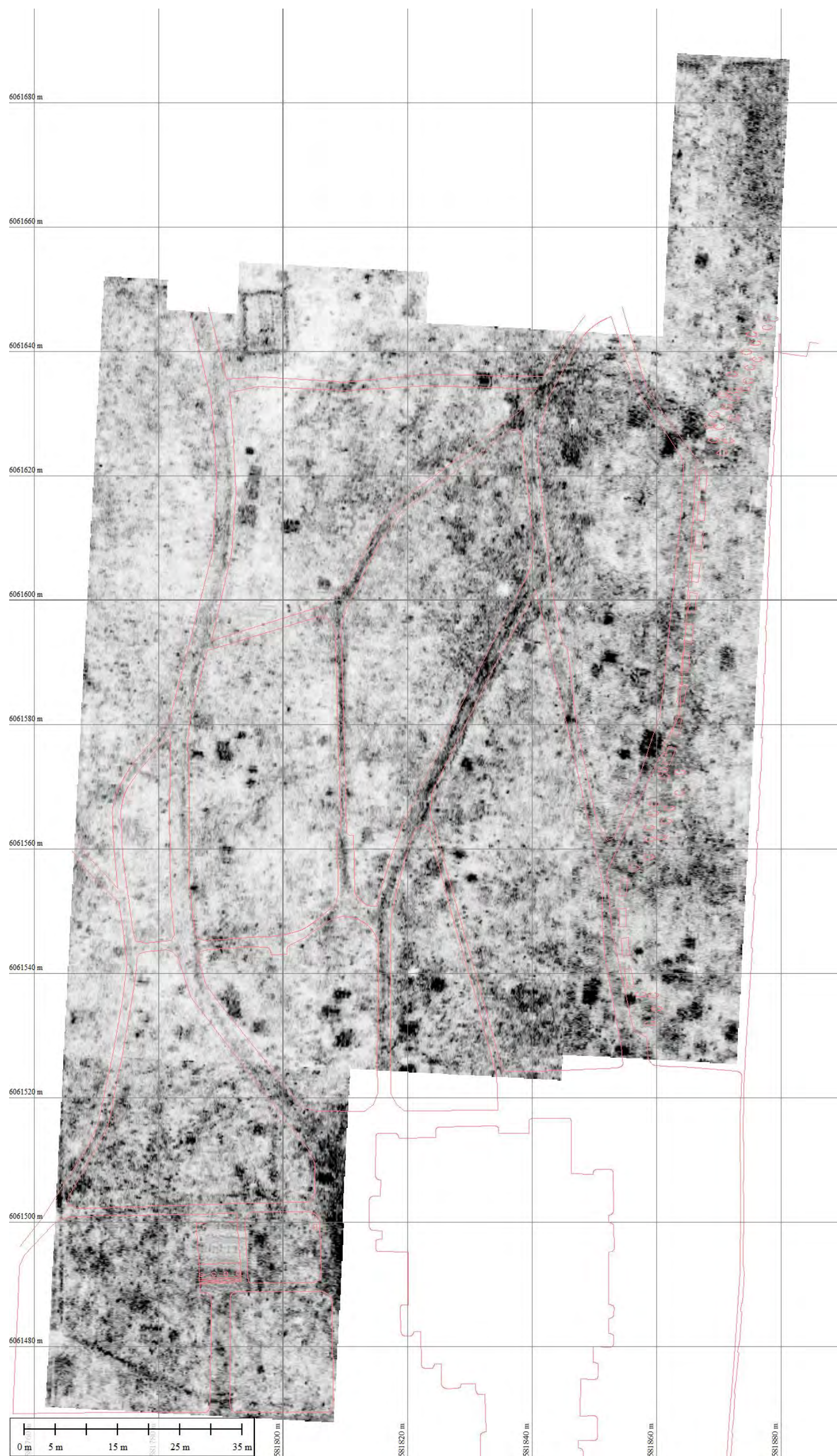
4 priedas. Suminis 10-20 ns anomalijų žemėlapis (60 – 120 cm gylio)
