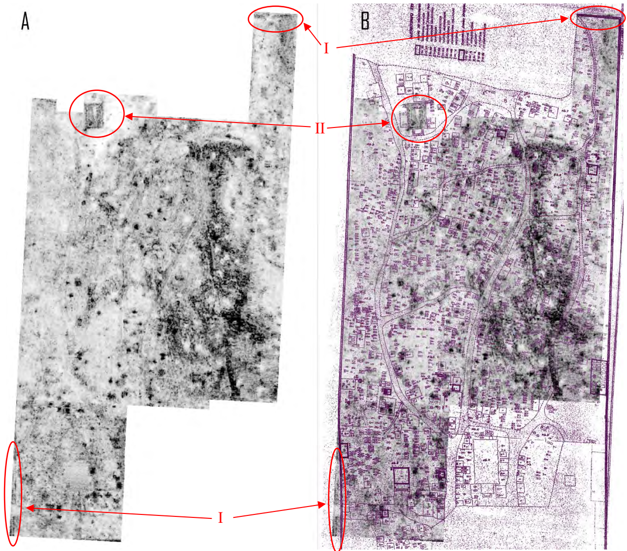
7 pav. Suminis 20-30 ns anomalijų žemėlapis (120 – 180 cm gylio). Sumuotas georadaro plokštuminis pjūvis (A), Suminis georadaro plokštuminis pjūvis su senu kapinių planą (B), raudona spalva pažymėtos anomalijos.
