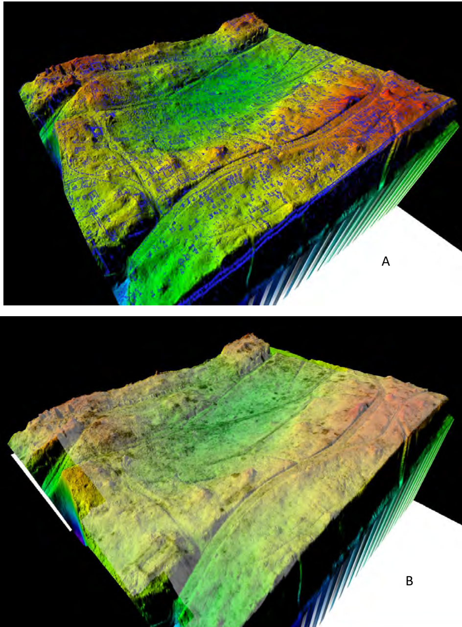
3 pav. Erdvinis paviršiaus reljefo vaizdavimas perdengiant jį senuoju kapinių planu (A) bei georadaro anomalijų žemėlapiu (B)
