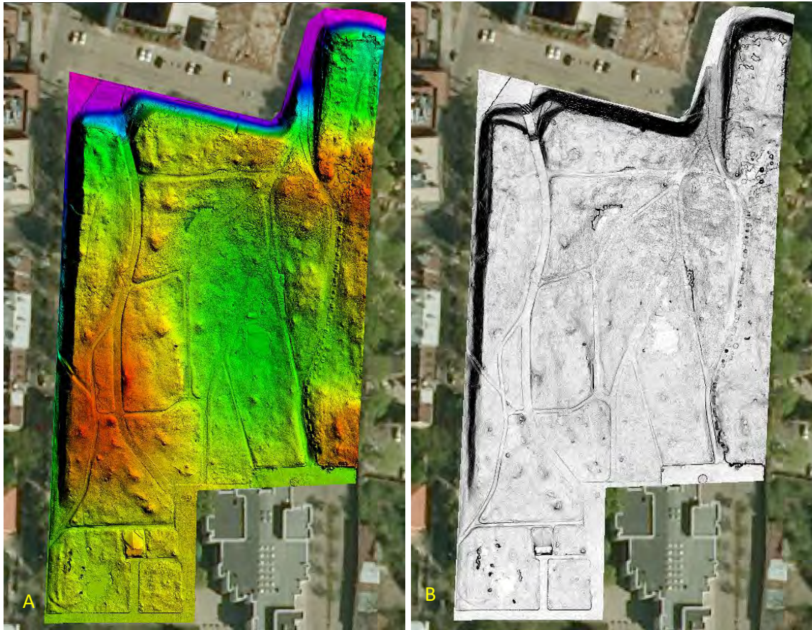
2 pav. Paviršiaus reljefo vaizdavimas spalvinėje skalėje (A) bei šlaitų statumo skalėje (B)
