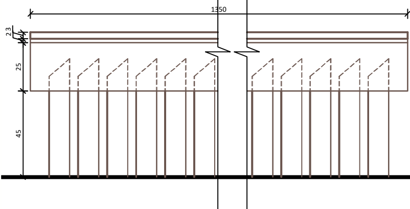
SKERSINIS PJŪVIS M 1:20
