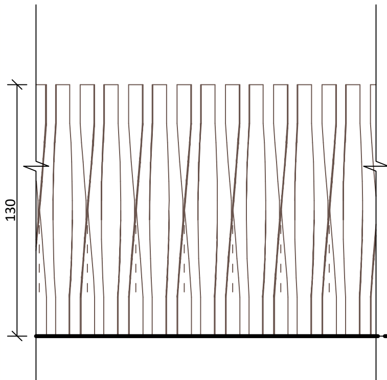
TVOROS SEGMENTO VAIZDAS IŠ PRIEKIO M 1:20
