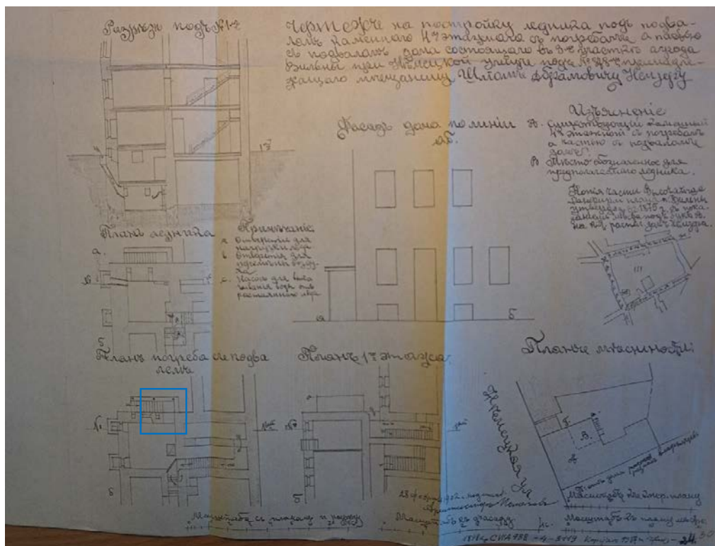
10/12a pav. Vokiečių g. 12 namo, 1902 m. projektas, kuriame numatyta buvusio rūšio vietoje įrengti rūši-ledainę. Mėlynai pažymėta 2021 m. tyrimų metu šurfe nr. 14 rastų struktūrų vieta, atitinkanti buvusio įėjimo į rūšį vietą. Planas paimtas iš VAA, F. 1019, ap. 11, b. 7655, l. 30
