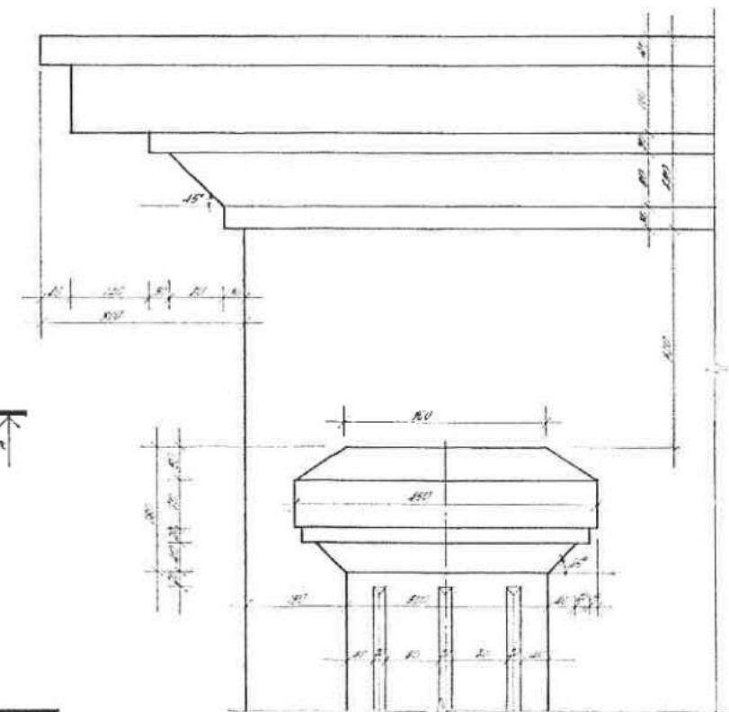
DETALĖ "2" M 1:5
