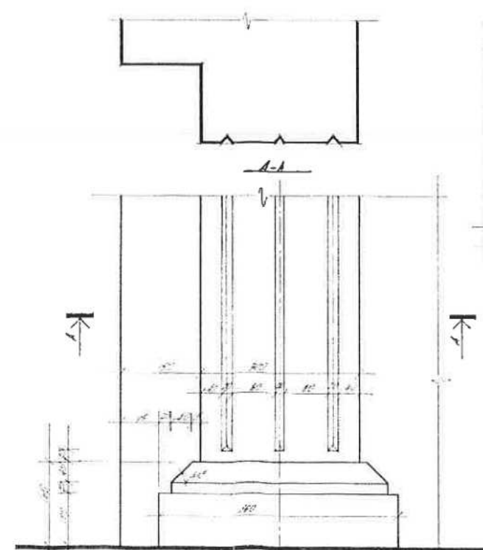
DETALĖ "1" M 1:5
