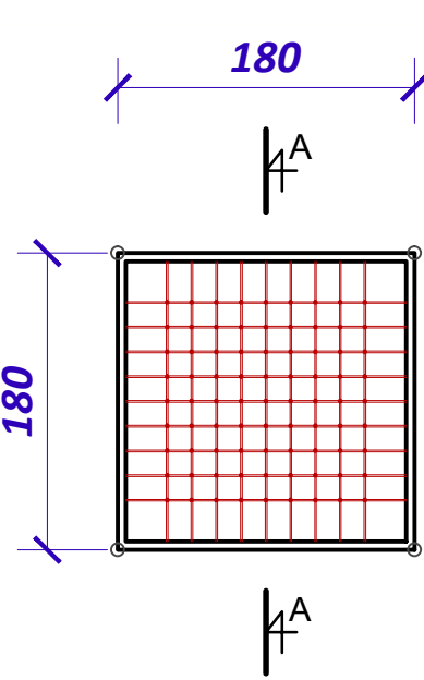
A tipo tinklo planas M 1:50
