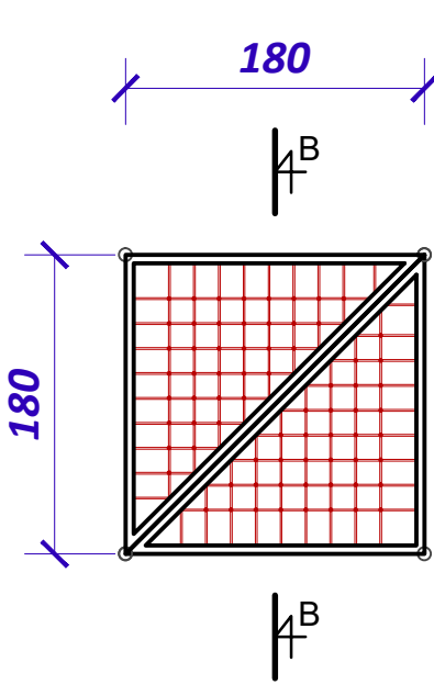
B tipo tinklo planas M 1:50
