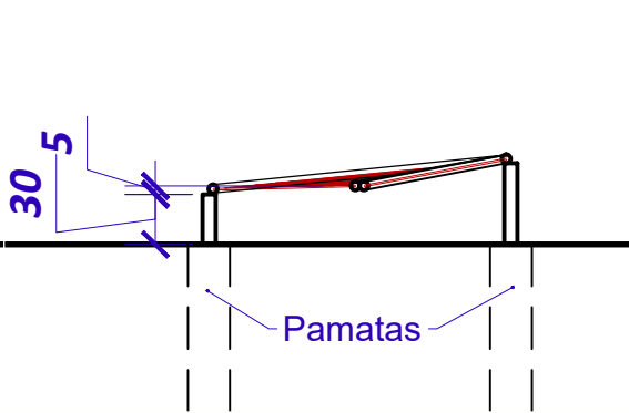
Skersinis pjūvis B-B M 1:50
